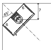
HWAM 5530
